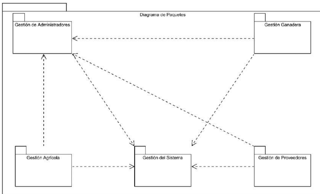
Figura 16. Diagrama de paquetes del sistema. Elaboración Propia
